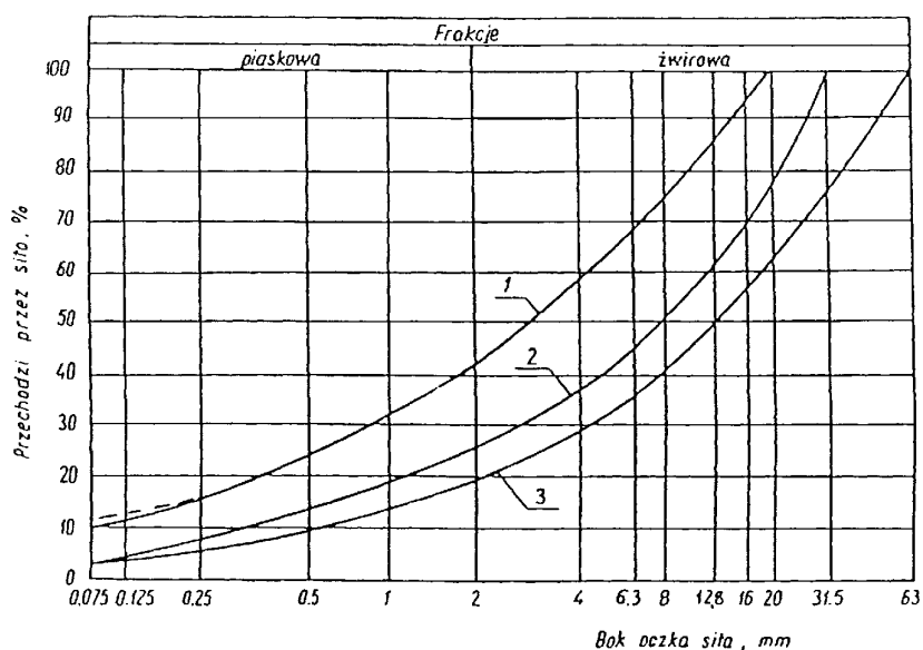
Rysunek 1. Pole dobrego uziarnienia kruszywa przeznaczonych na podbudowę
